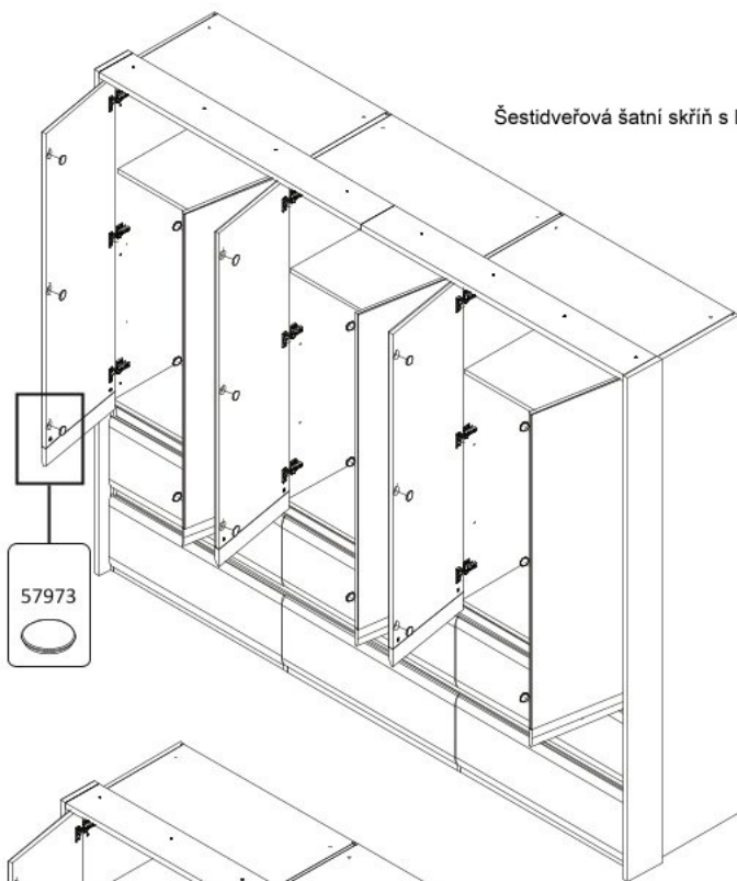
Šestidveřová šatní skříň se 2 zrcady a LED osvětlením
